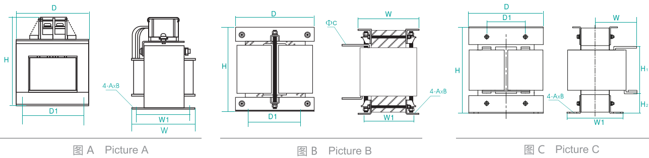
380V输入直流电抗器选型表 380V Input DC Reactor Selection Table
